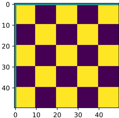
Cosine
